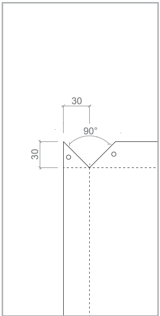
DETALLE B
