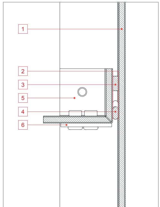
DETALLE DE FIJACIÓN MECÁNICA
