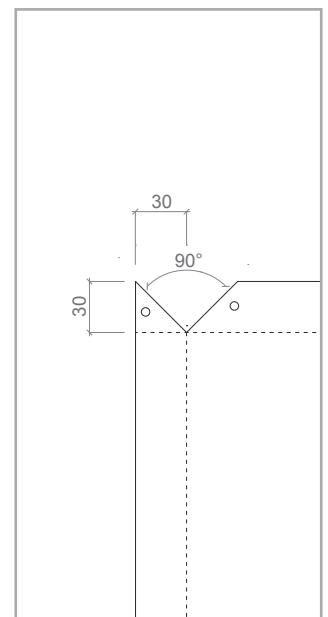
DETALLE B
