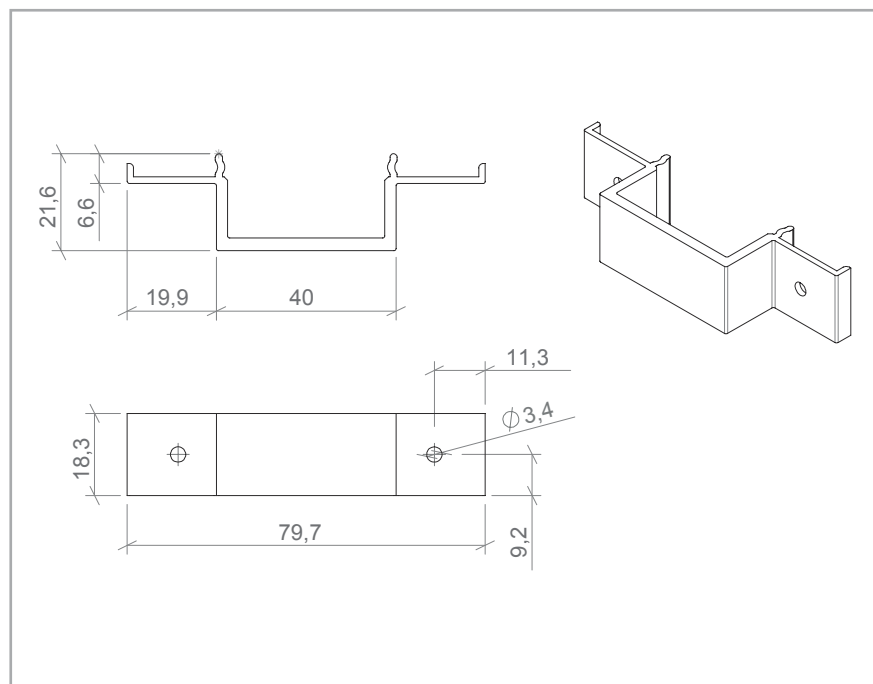
SOPORTE CUELGUE STB-T-CH
