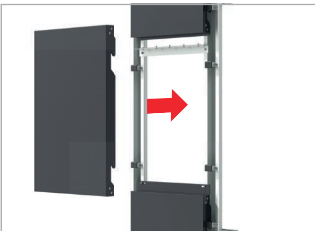
5. Colocación de la nueva bandeja de panel composite STACBOND® , con bota de cuelgue especial de 9 mm y piezas de refuerzo de cuelgue.
